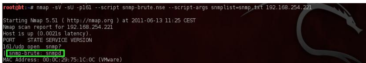
Figura 101: Script NSE snmp-brute
