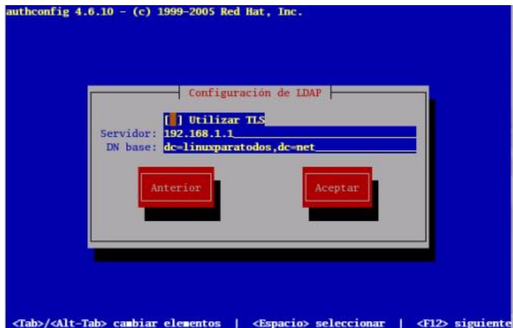
authconfig, pantalla configuración ldap.
