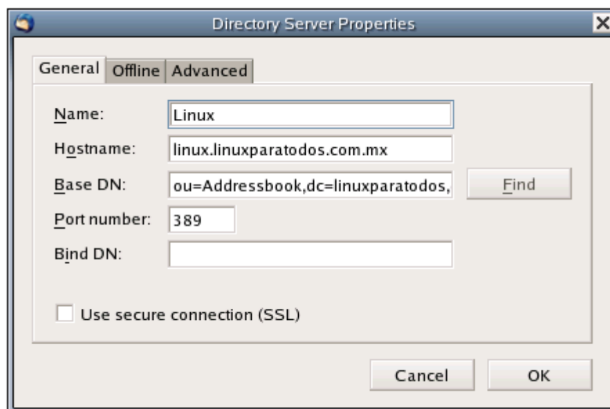
Propiedades de servidor de directorio, pestaña General.
