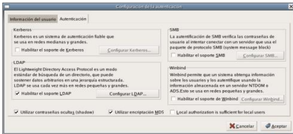
authconfig-gtk, pestaña de Autenticación.
