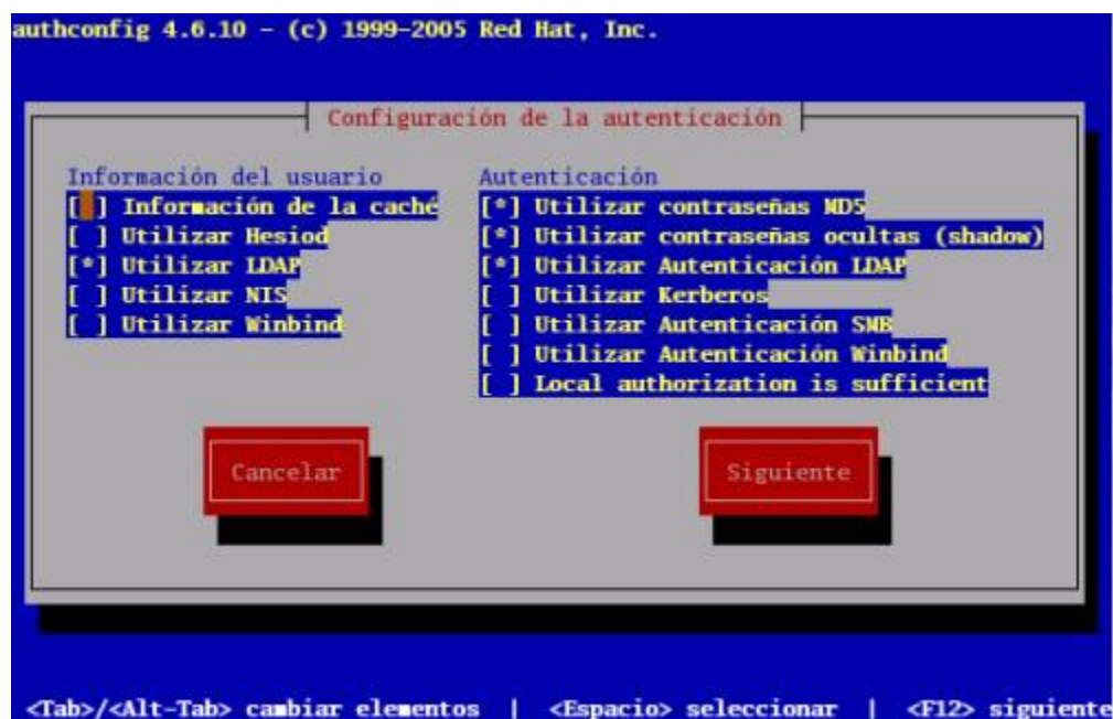
uthconfig, pantalla principal.
