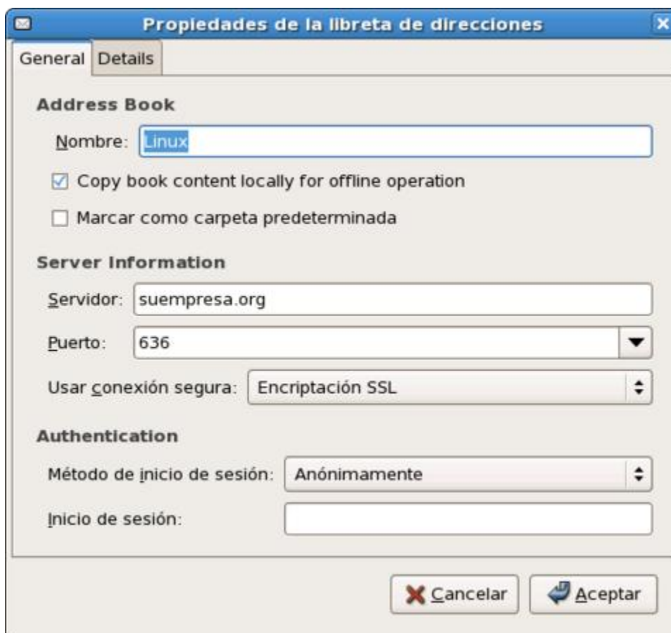
Configuración LDAP, GNOME Evolution.
