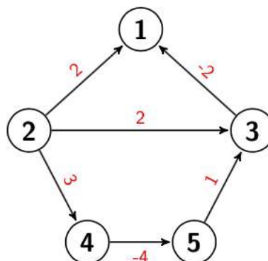
Imatge 34. Graf amb arestes amb valors negatius. Imatge extreta de https://aprende.olimpiada-informatica.org/algoritmia-dijkstra-bellman-ford-floyd-warshall
