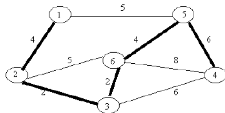
Imatge 10. La línia fosca és l'arbre d'expansió del graf. Imatge extreta de https://users.dcc.uchile.cl/~raparedel/clases/cc30a/00.2/tarea3/tarea3.html
